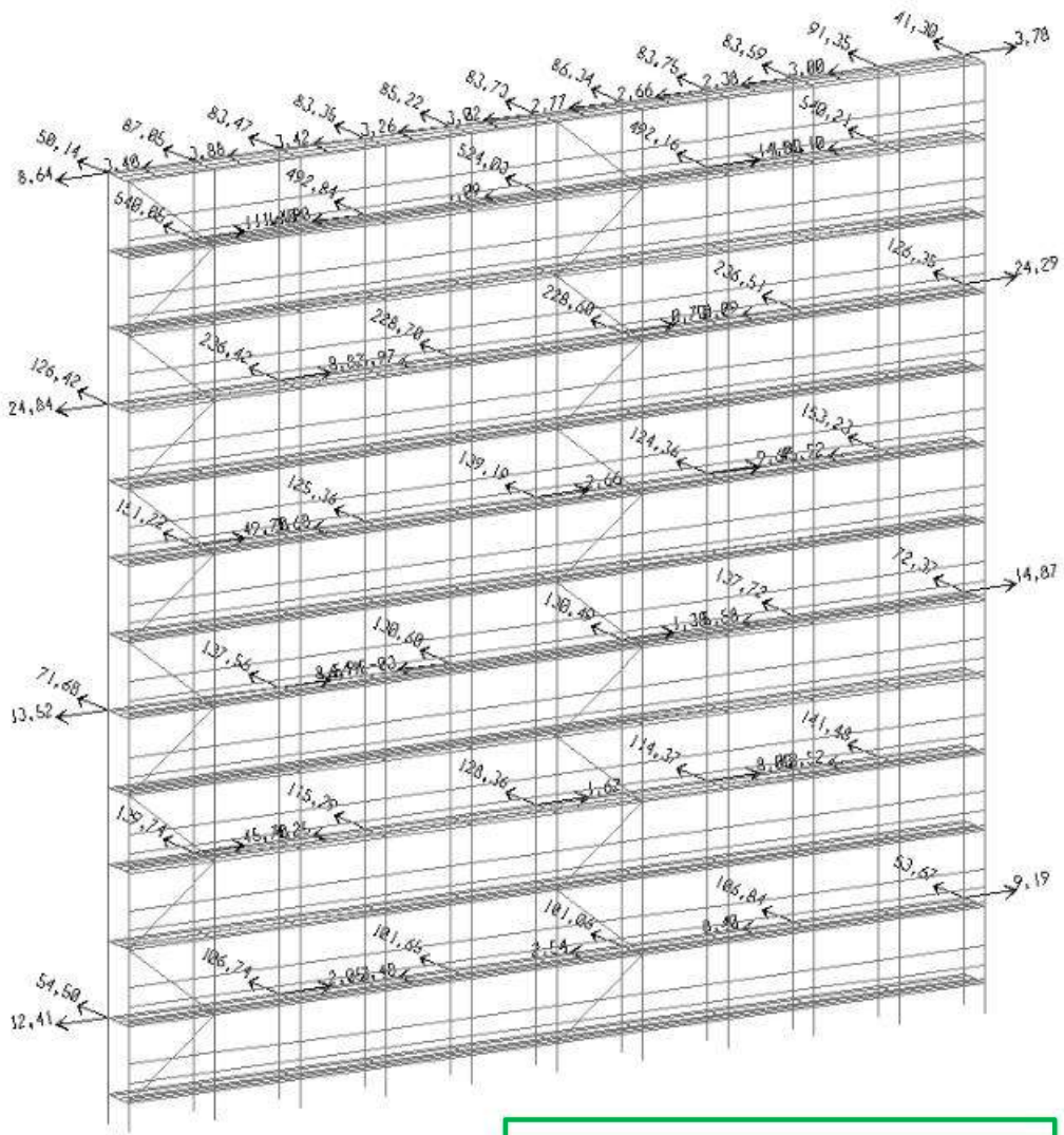
Şekil 9.1: Envelope kombinasyonuna göre ankraj kuvvetleri (ton,m )
