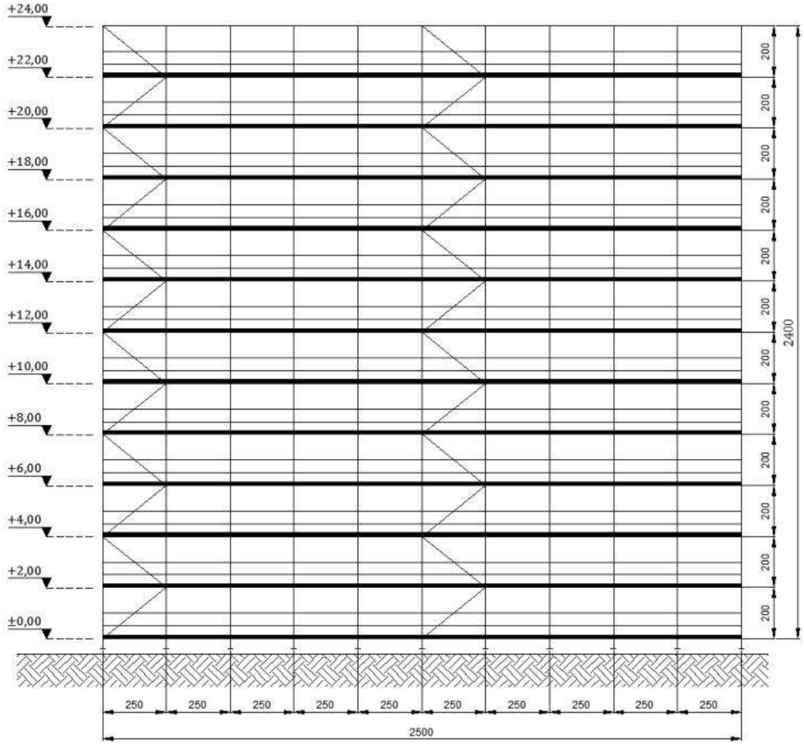
Şekil 3.1 : 25,0 metrelik cephe görünümü
