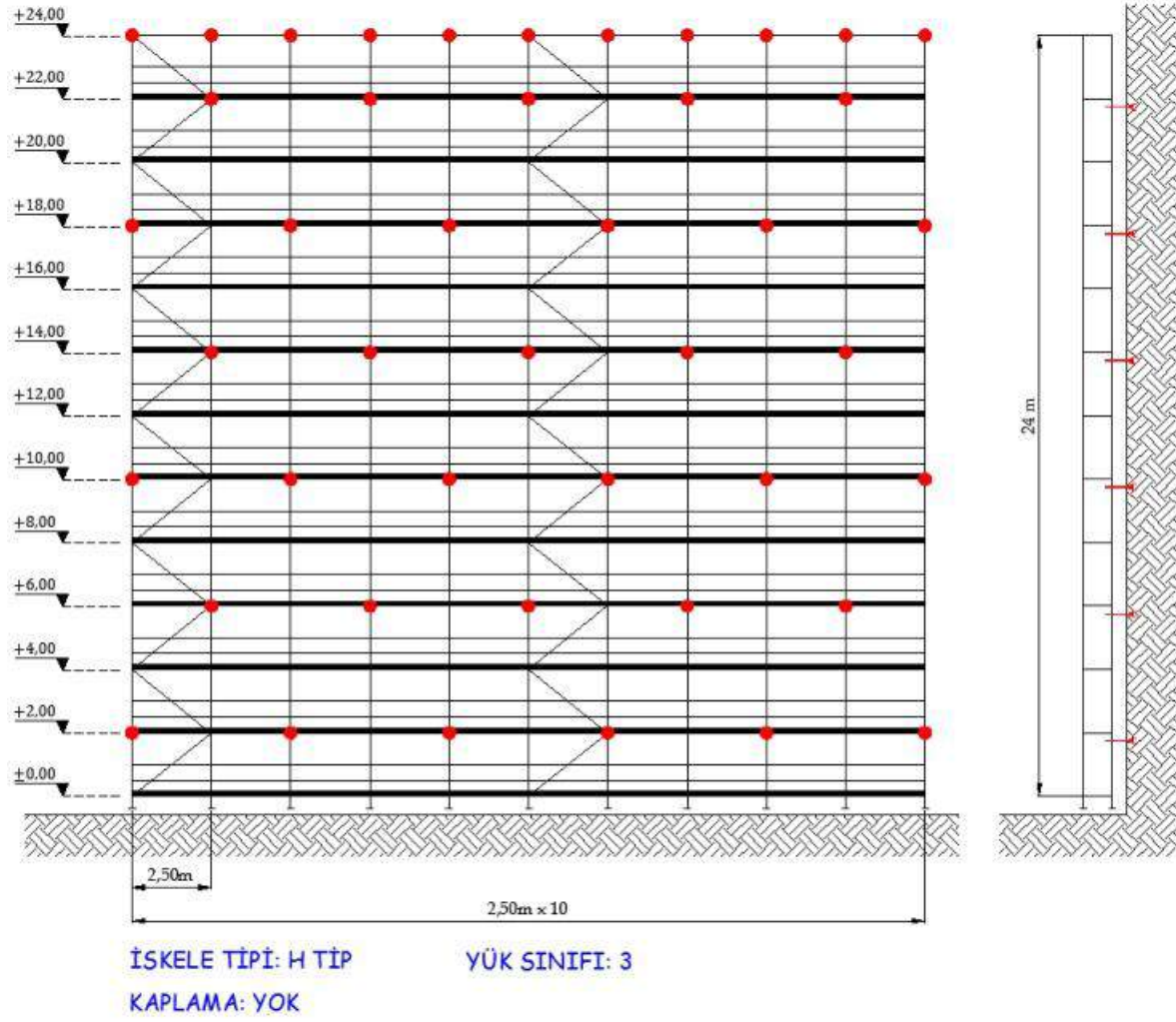
Şekil 3.2 : Ankraj Konfigürasyonu
