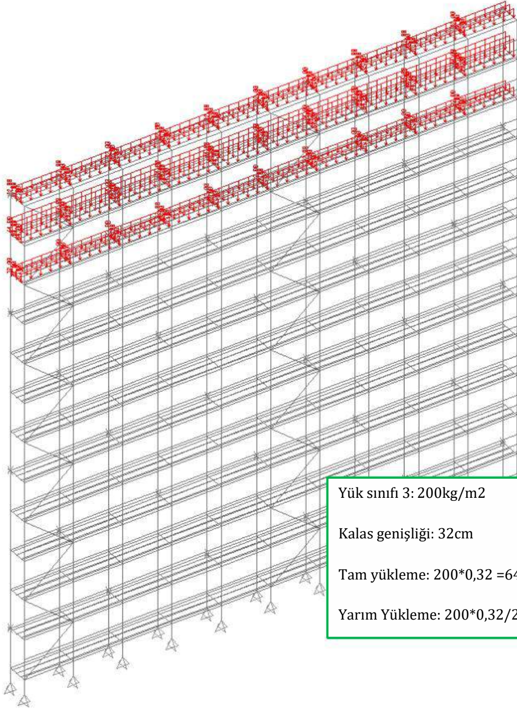
Şekil 7.1: Hareketli yükler
