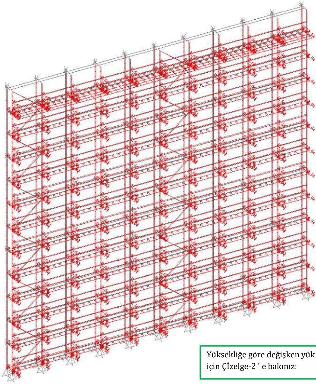
Şekil 7.5: WdikH Yükleme (kg/m) (hizmet)
