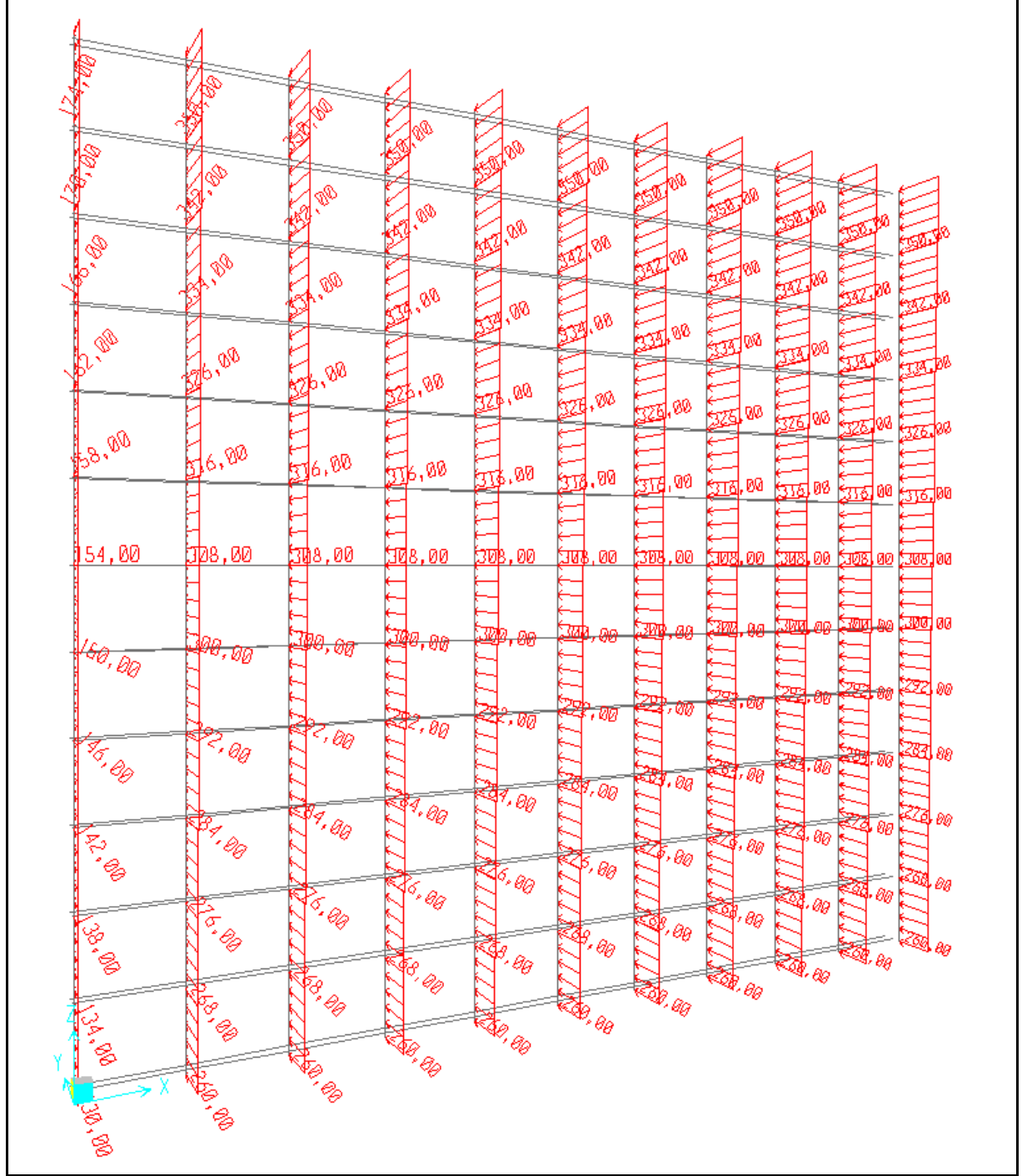
Şekil 7.2: Dikmelerde Wdik Yükleme (kg/m)
