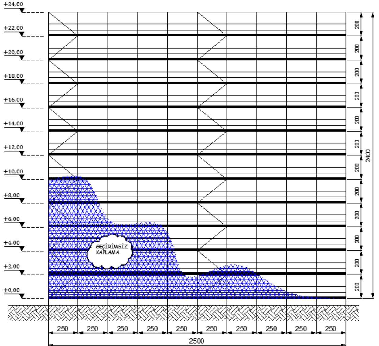
Şekil 3.1 : 25,0 metrelik cephe görünümü
