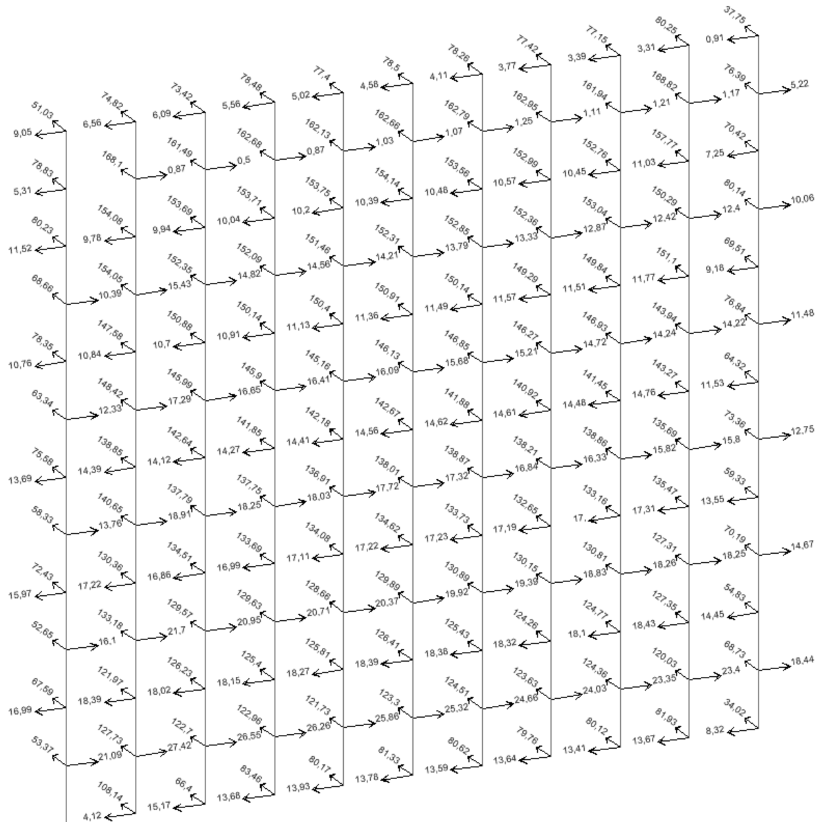
Şekil 9.3: Kombinasyon 3' e göre mesnet tepki kuvvetleri ( kg,m )
