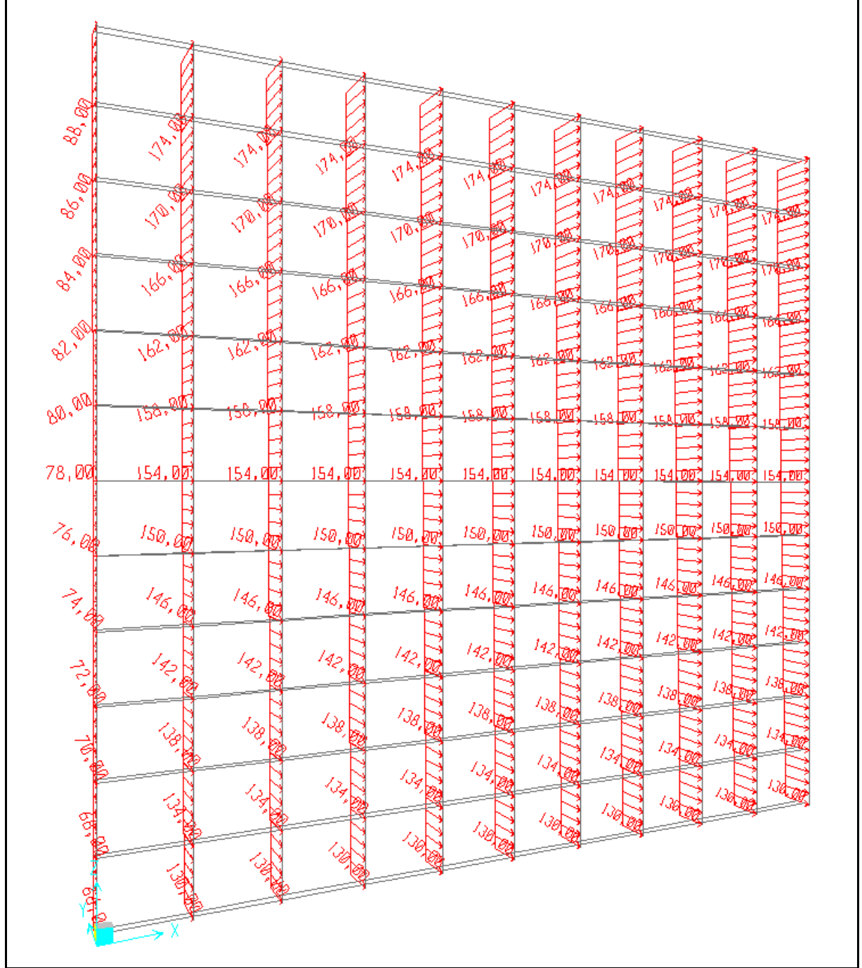
Şekil 7.3: Dikmelerde -Wdik Yüklemesi (kg/m)
