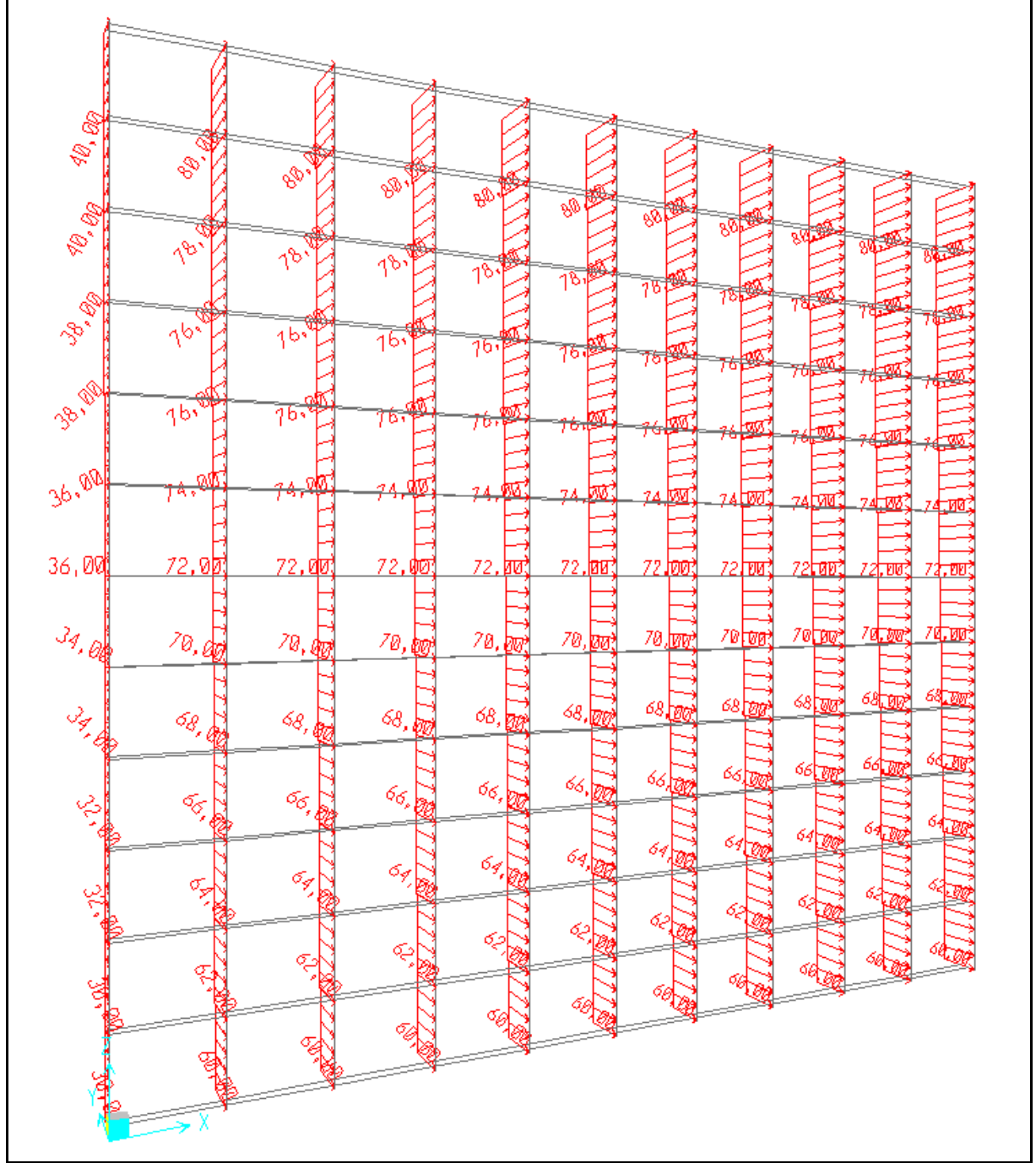
Şekil 7.4: Dikmelerde Wparalel Yüklemesi (kg/m)
